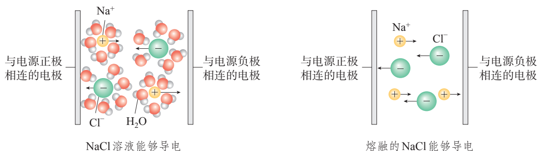
图 1-12 NaCl 导电示意图
