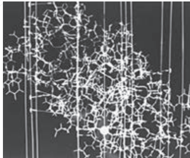
牛胰岛素分子结构模型
