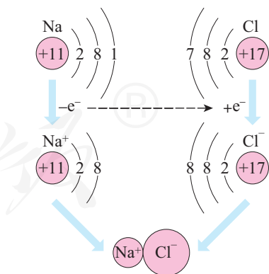
图 1-13 NaCl 的形成示意图
