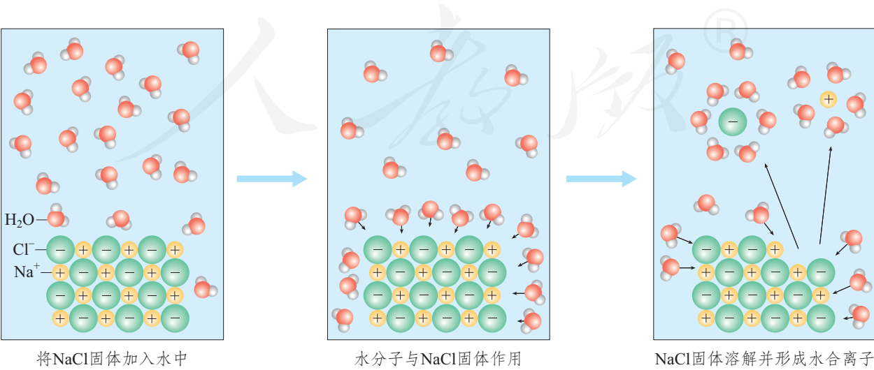
图1-11 \text{NaCl} 固体在水中的溶解和形成水合离子示意图
